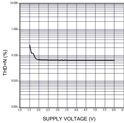
总谐波失真 vs. 供给电压
