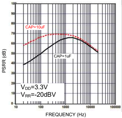
电源纹波拒斥比 vs. 频率
