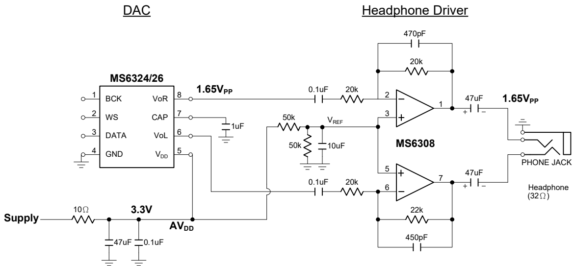
图五、数字转模拟输出一阶低通滤波器。
