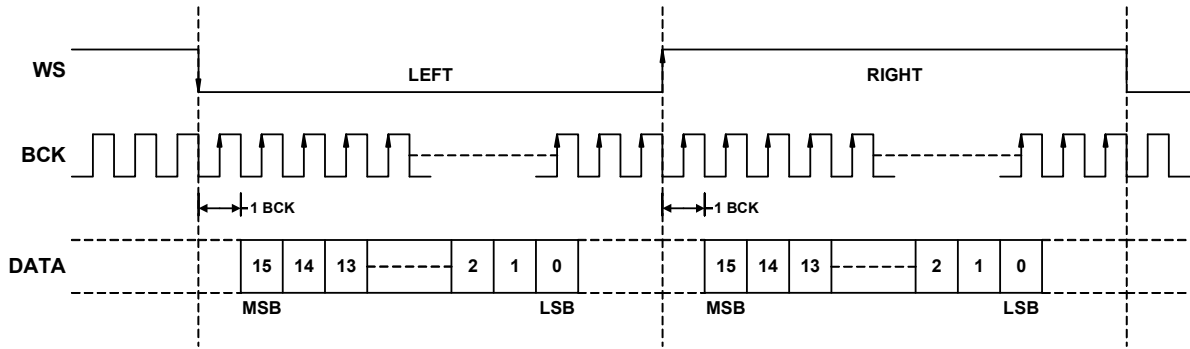
图四、输入信号格式I 2 S (MS6324)
