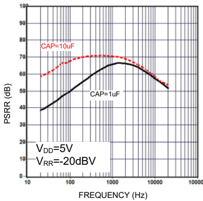
电源纹波拒斥比 vs. 频率
