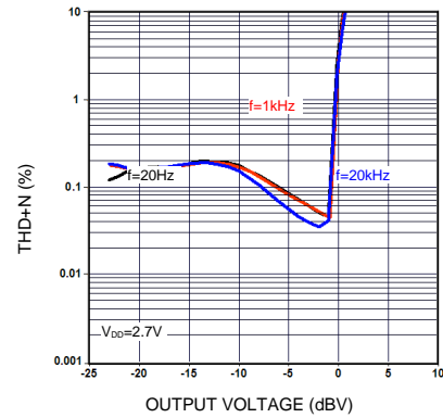
THD+N vs. 输出电压(2.7V)
