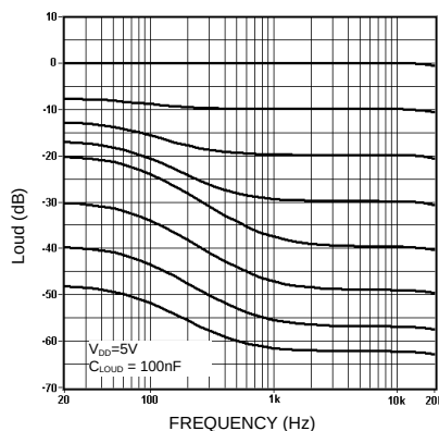
響度 VS. 頻率 VS. 音量
