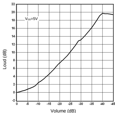
響度 VS. 音量
