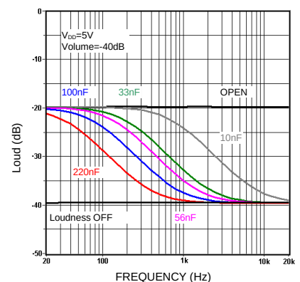
響度 VS. 外部電容
