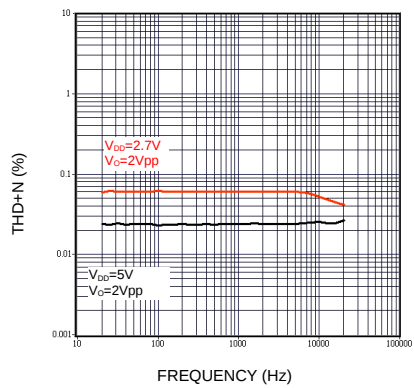
THD+N vs. 頻率
