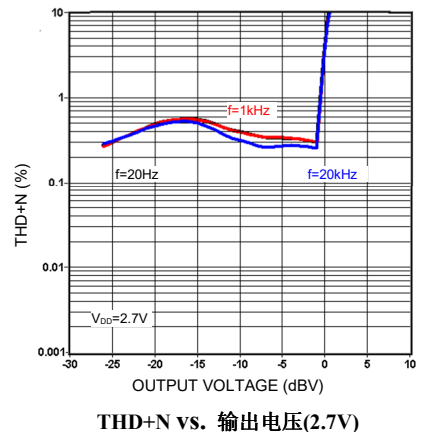
THD+N vs. 输出电压(2.7V)
