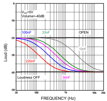
響度 vs. 外部電容
