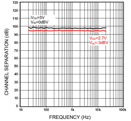
声道隔离度 vs. 频率
