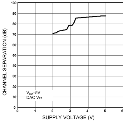
聲道隔離度 vs. 電壓
