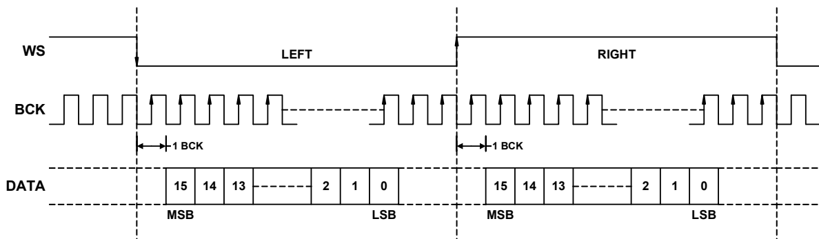
圖四、輸入信號格式 (I 2 S)
