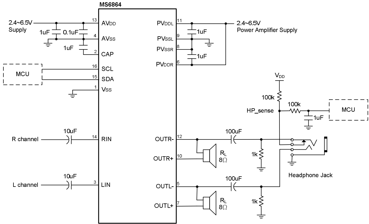
圖五、基本應用電路
