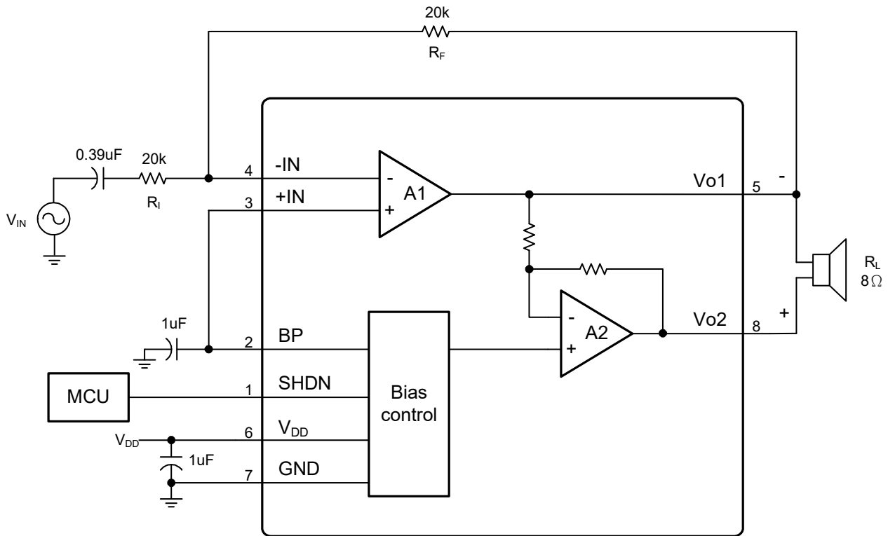
圖一 音頻放大器應用電路
