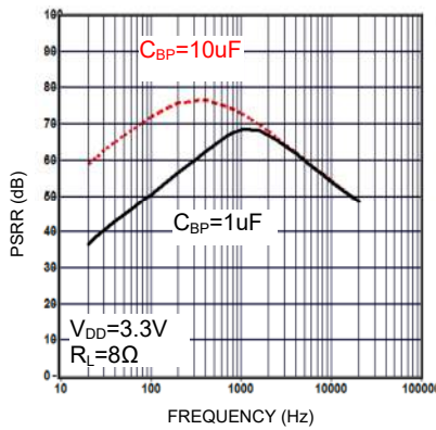
PSRR vs. 頻率
